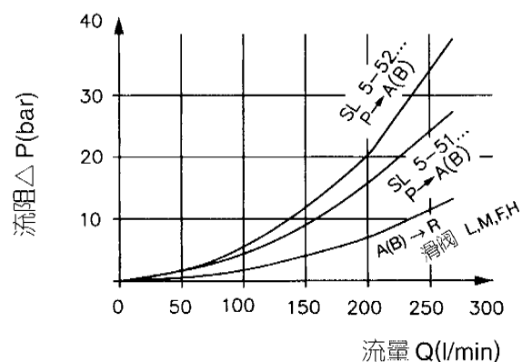
滑阀 流阻 (全行程)
