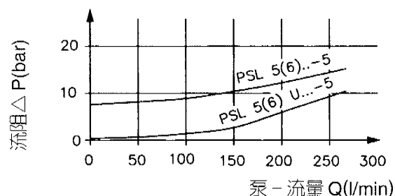
滑阀 流阻 (全行程)
