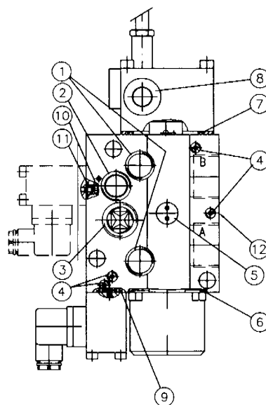
多路阀 (滑阀)
