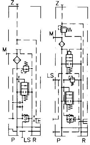
PSL5(6)/... PSL5(6)U/... PSL5(6)UH/...
