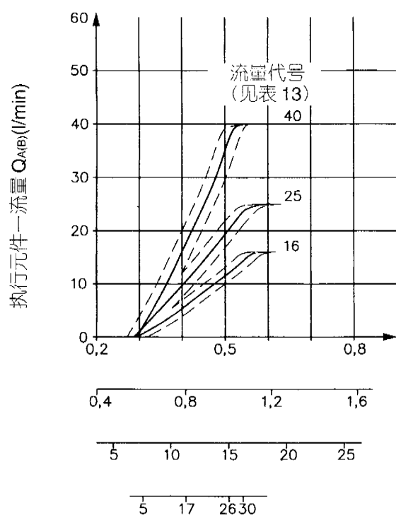
滑阀 控制曲线
