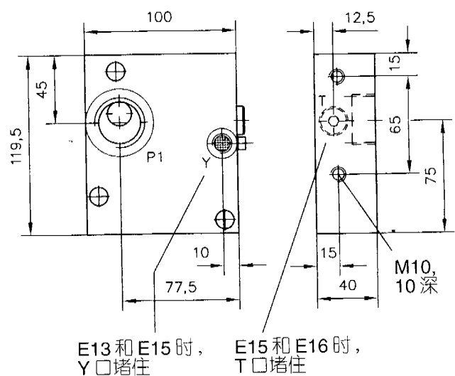
终端块 E13 至 E16
