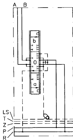
4/3- 换向滑阀 无进口流量调节阀 ..1...
