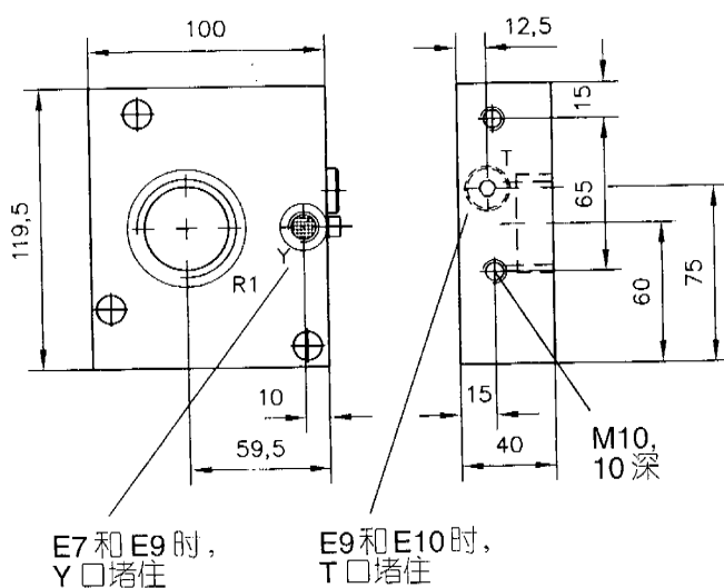
终端块 E7 至 E10
